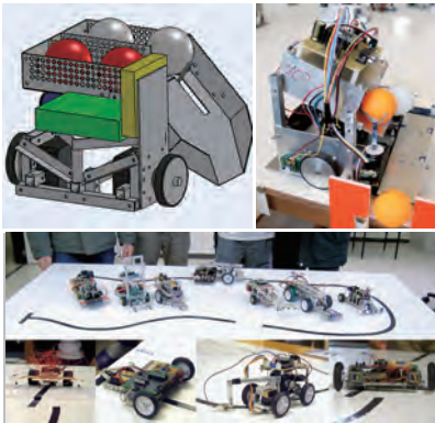
PBL実験で使用したロボット Robots made by PBL experiment
